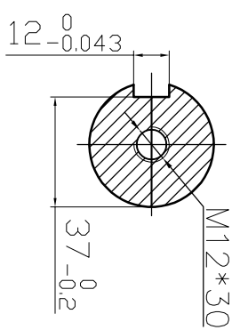
A-A(2:1)
